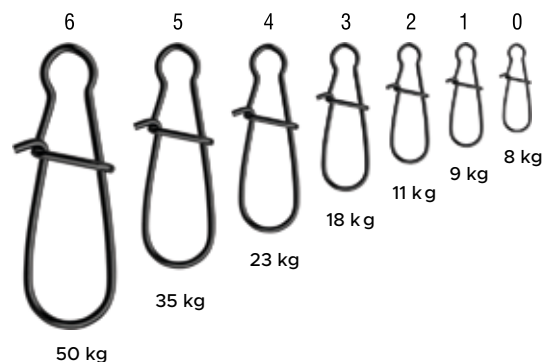
572004 FASTLOCK SNAP V K-2175
