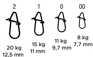
572004 FASTLOCK SNAP V K-2175
